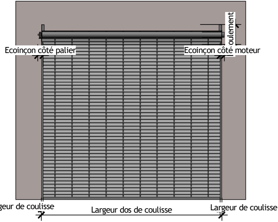
5 Elévation Arrière Ech : 1 : 50
