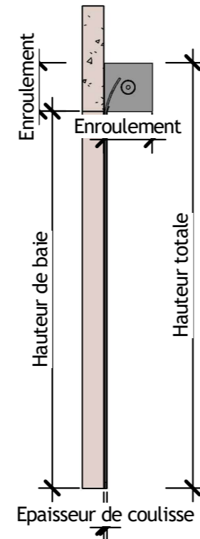
2 Vue en coupe Ech : 1 : 50
