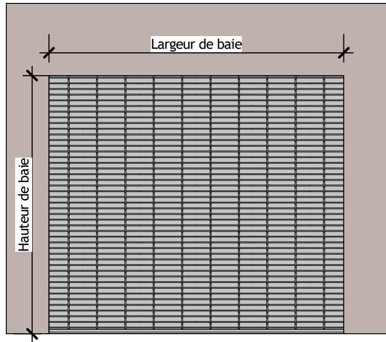
4 Elévation Avant Ech : 1 : 50
