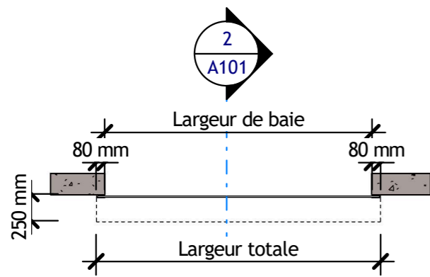
1 Niveau 0 Ech : 1 : 50
