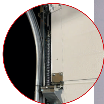
Ressorts de traction dans les montants
